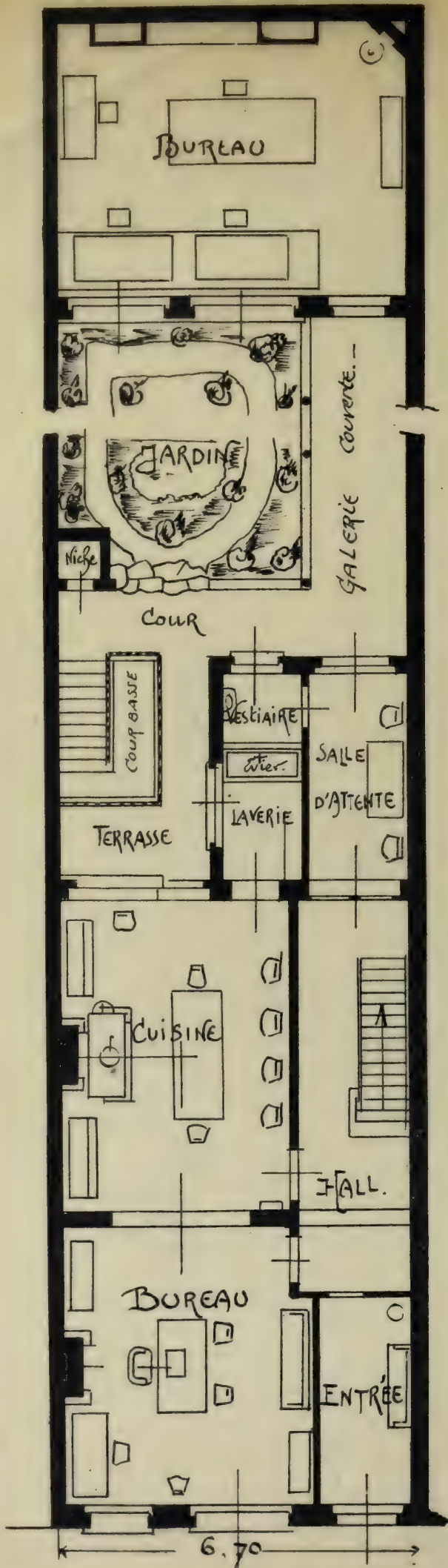
REZ-DE-CHAUSSÉE
